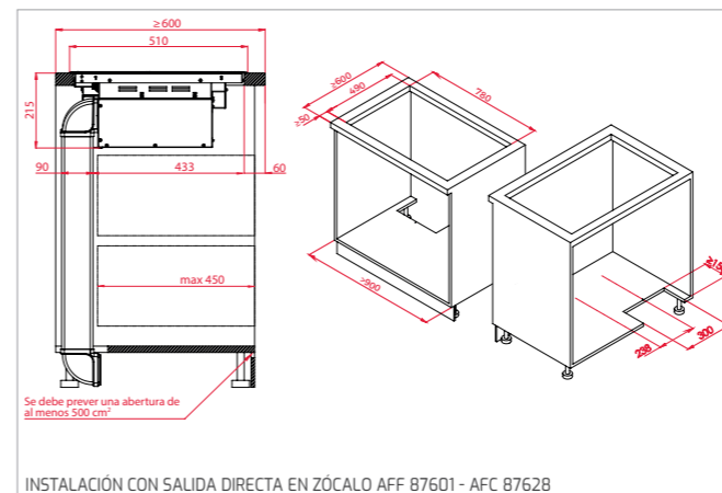
INSTALACIÓN CON SALIDA DIRECTA EN ZÓCALO AFF 87601 - AFC 87628
