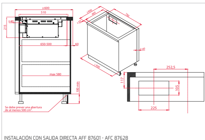
INSTALACIÓN CON SALIDA DIRECTA AFF 87601 - AFC 87628
